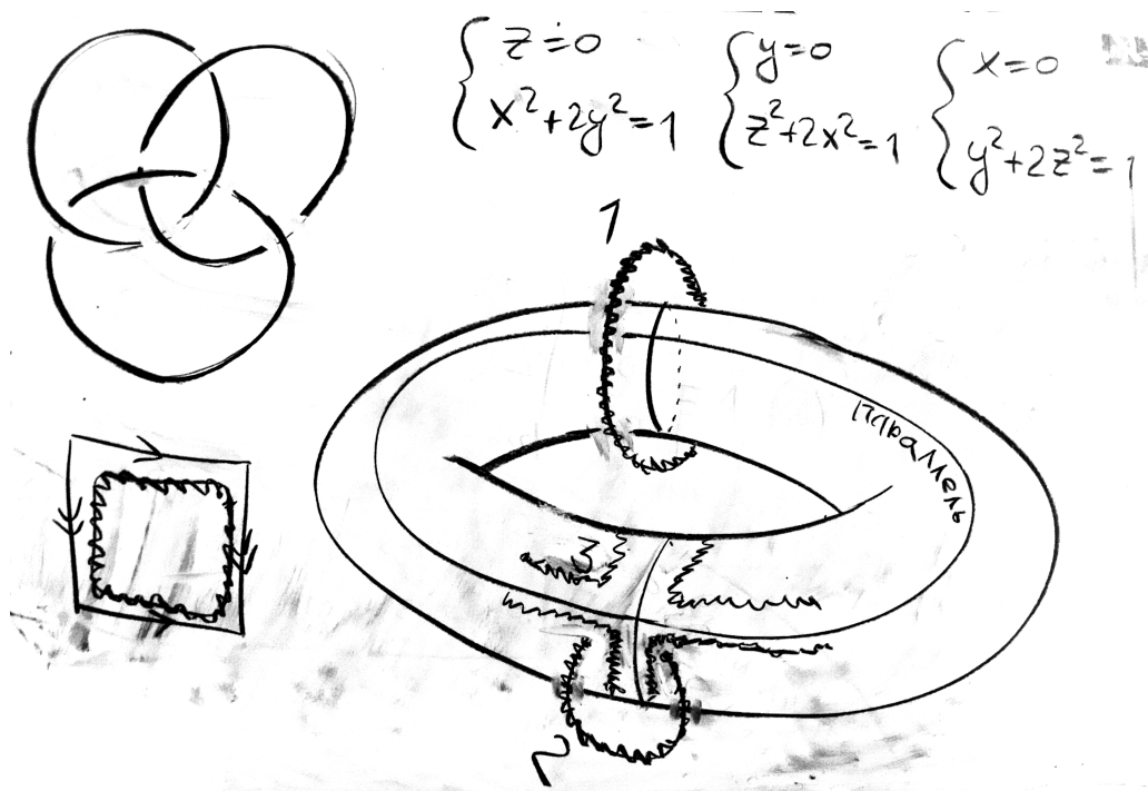
Рис. 1: Три lika колец Борромео
