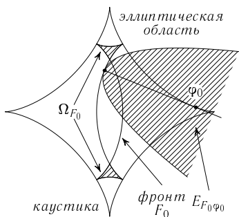
Рис. 23. Треугольники гиперболичности
