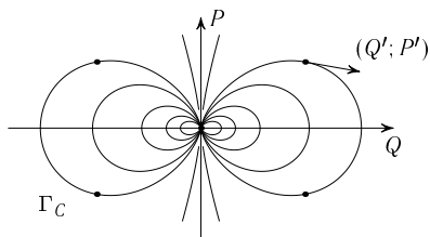
Рис. 11. D -критические кривые
