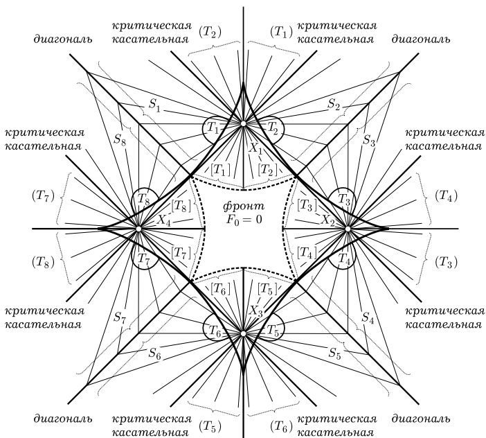
Рис. 25. Заметание эллиптической области отрезками
