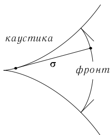
Рис. 26. Построение (гипер)фронта
