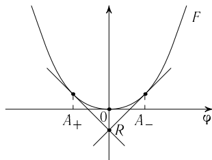
Рис. 16. Огиперболичивание
