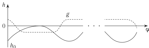
Рис. 9. Возмущение гессиана
