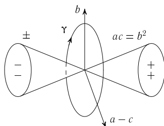
Рис. 3. Гиперболическая кривая индекса 1
