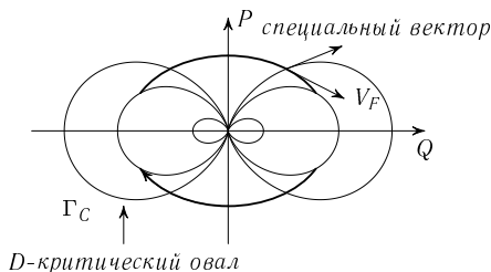
Рис. 12. D -гиперболичность как трансверсальность
