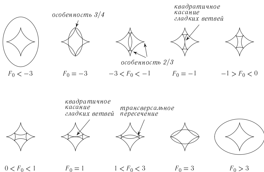
Рис. 21. Перестройки фронтов астроиды
