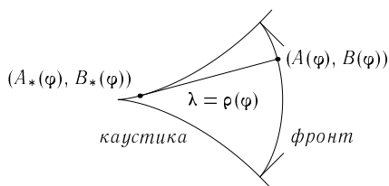
Рис. 2. Фронт как эвольвента каустики
