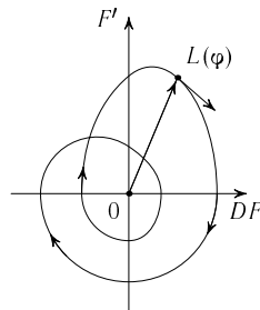
Рис. 10. Два оборота вокруг нуля
