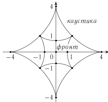
Рис. 1. Эвольвента астриды
