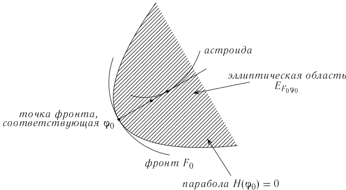
Рис. 22. Эллиптическая область
