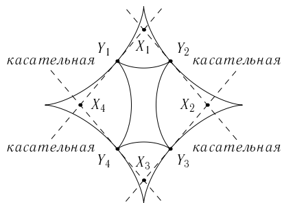
Рис. 24. 4 X -точки астроиды
