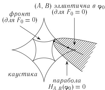
Рис. 20. Астроидальный 0-фронт
