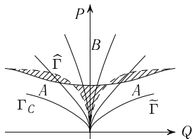
Рис. 13. А-деформация и В-деформация кривой \hat{\Gamma}
