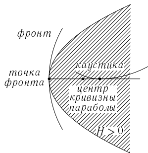
Рис. 19. Парабола, ограничивающая область эллиптичности
