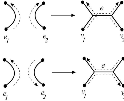
Рис. 8. Два пути
