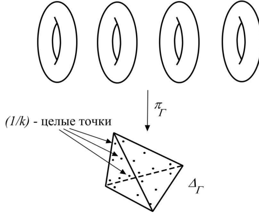
Рис. 5. Поляризация Голдмана
