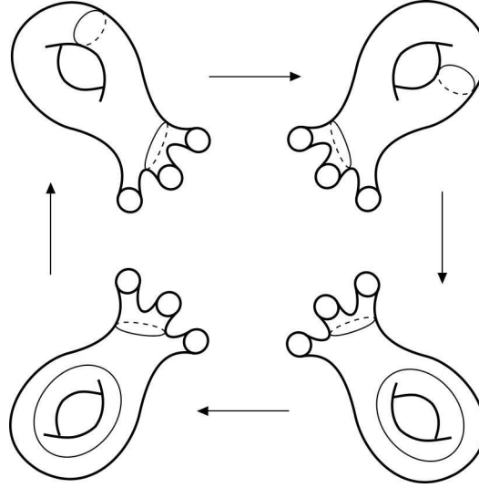
Рис. 11. Четырехугольники
