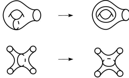
Рис. 7. Элементарные преобразования
