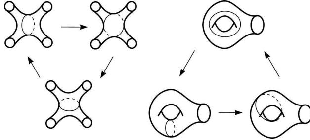
Рис. 10. Треугольники
