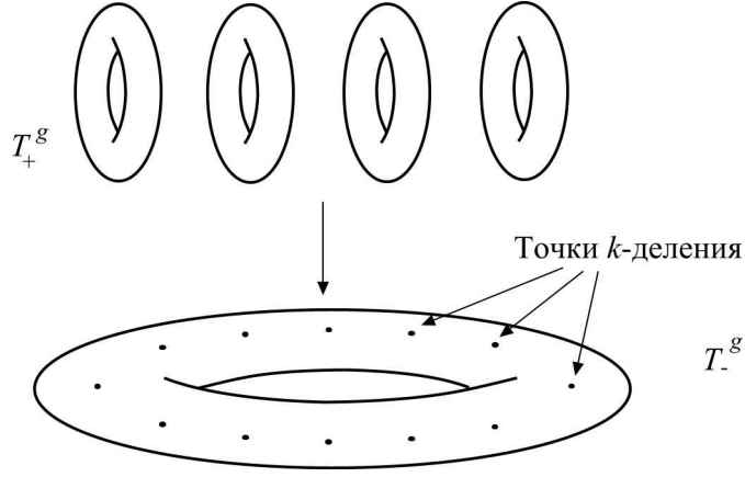
Рис. 2. Бор-зоммерфельдовы точки тора
