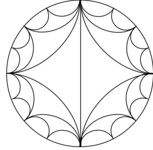
Рис. 9. Граф Фарей.
