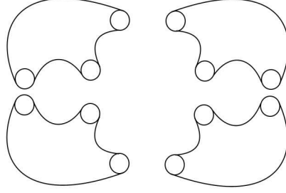
Рис. 4. Раскрой на штаны
