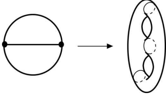
Рис. 6. Утолщение графа.
