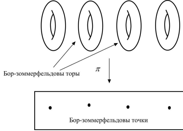
Рис. 1. Бор-зоммерфельдовы слои
