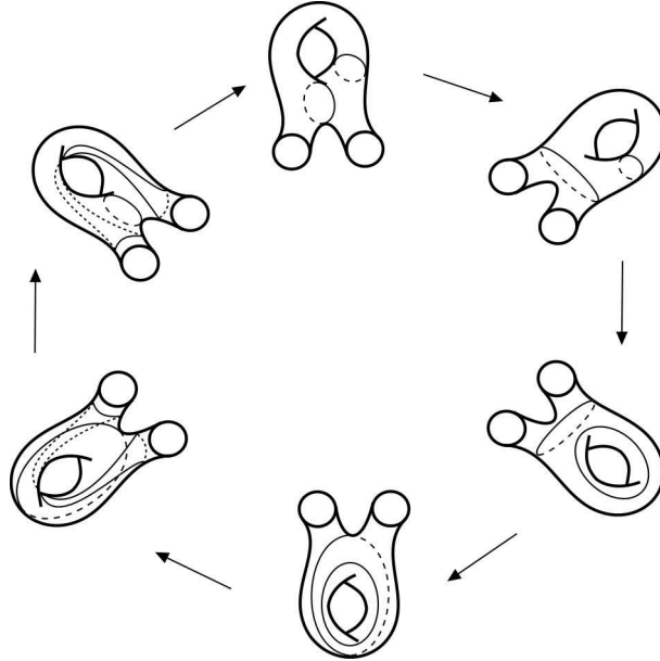
Рис. 13. Шестиугольники
