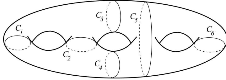
Рис. 3. Полный набор простых петель
