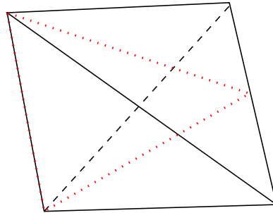
Симплекс разбит в объединение двух симплексов одинакового объема
