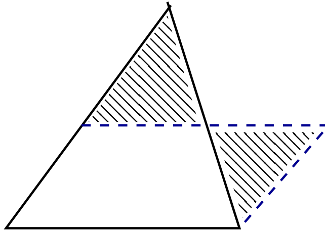
Любой треугольник равносоставлен параллелограмму с тем же основанием и одним из углов.
