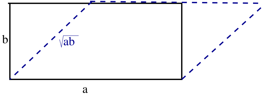
Прямоугольник со сторонами a > b равносоставлен параллелограмму со сторонами a и \sqrt{ab} .
